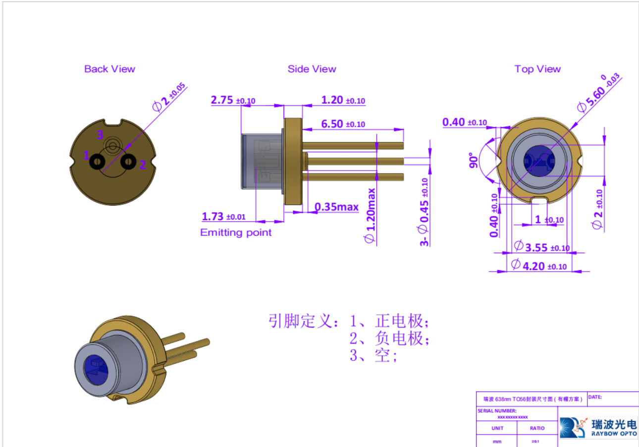
三引脚尺寸图
